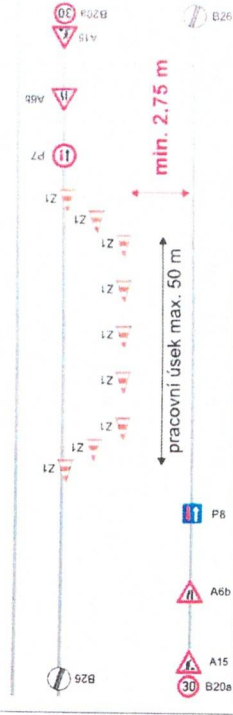
VZOR č.4 - krátkodobý (mobilní) zábor komunikace
